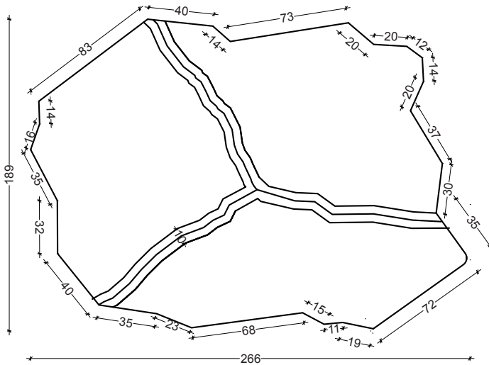
Plan (Scale :- 1 : 1.5)
