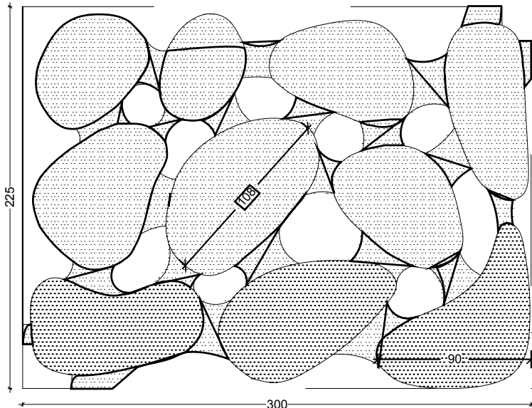
Plan (Scale :- 1 : 1.5)
